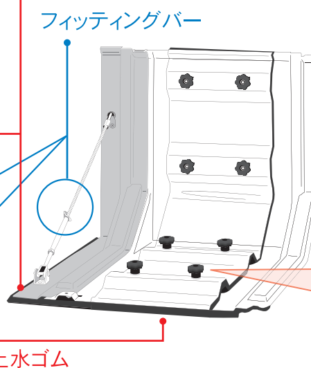
FSサイドシール + FT50
