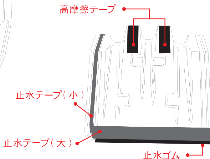
FZ平面止水板（底面）
